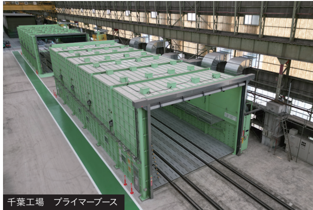
千葉工場 プライマーブース
